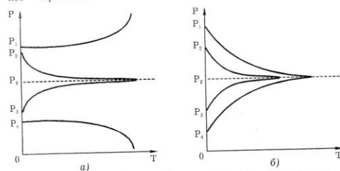
Рис. 3—17. Локальная (а) и глобальная (б) устойчивость равновесия
