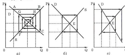
Рис. 3—19. Устойчивое (а) и неустойчивое (в) равновесие в паутинообразной модели и регулярные колебания (б) вокруг него
